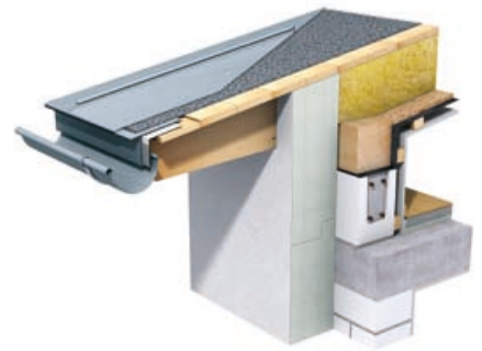
Fig. 2: Ikke-ventileret tagkonstruktion med fuld isolering af spærene
